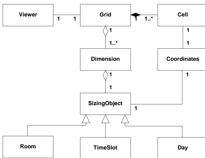
Figure 3.18 — Diagramme de classes du paquetage grid.
